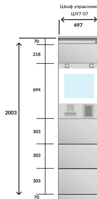
Шкаф управления без раздатчиков мешков и 4-мя ячейками выдачи
