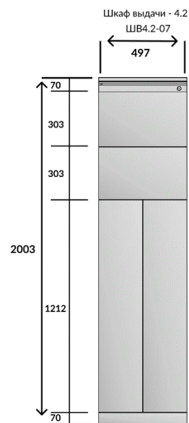
2 высокие + 2 низкие ячейки
