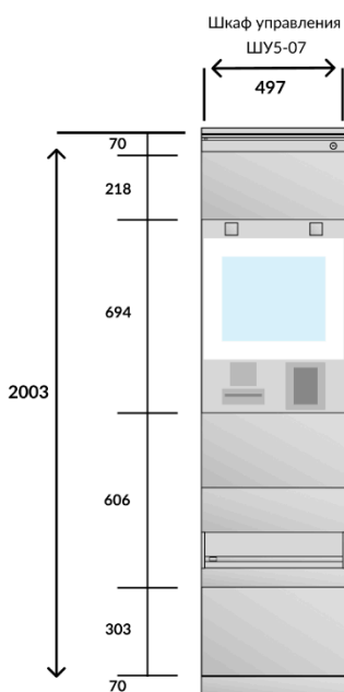
Шкаф управления с раздатчиками мешков и 2-мя ячейками выдачи
