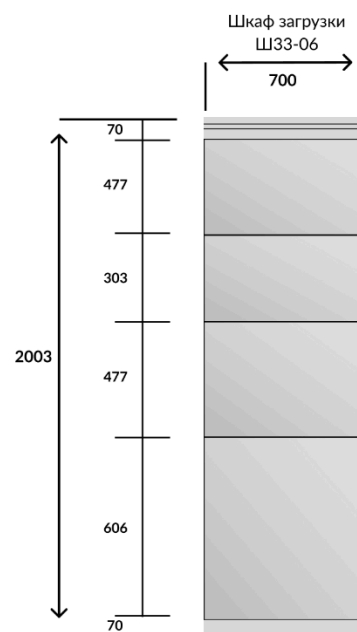
Шкаф загрузки с одной ячейкой выдачи
