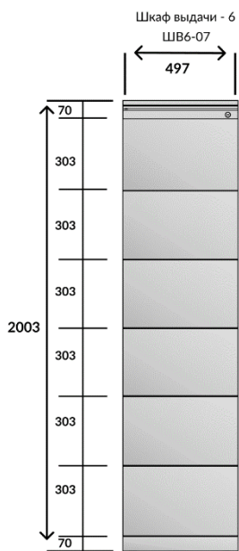
6 низких ячеек
