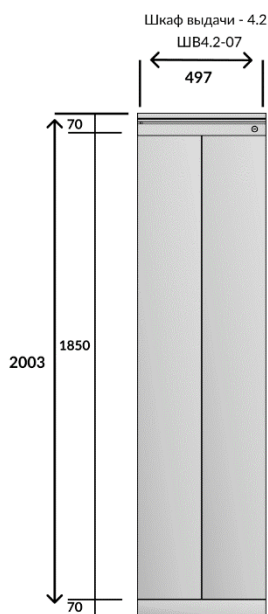
2 высокие ячейки
