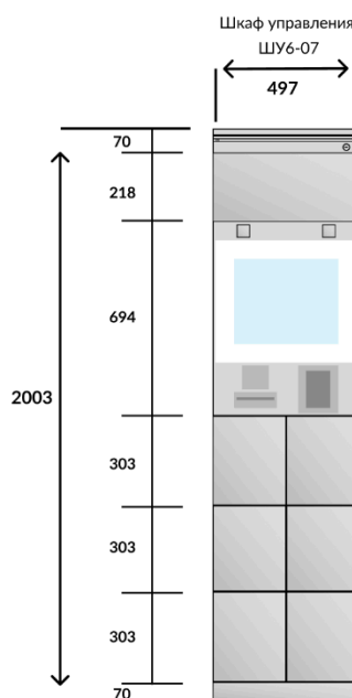
Шкаф управления без раздатчиков мешков и 10 ячейками выдачи (обувной)
